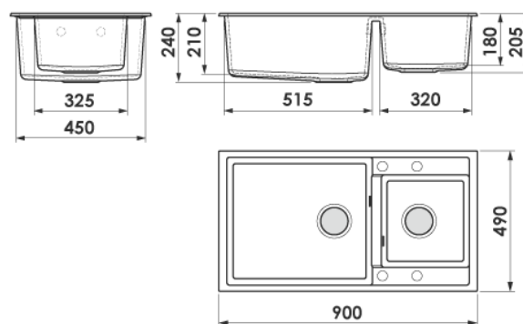
DVOUDŘEZ pravý / levý číslo modelu: 234 rozměr: 90cm x 49cm
