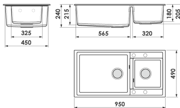
DVOUDŘEZ pravý / levý číslo modelu: 235 rozměr: 95cm x 49cm
