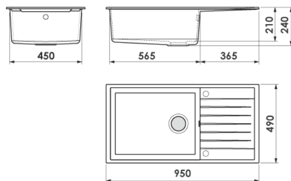
DŘEZ S ODKAPEM pravý / levý číslo modelu: 230 rozměr: 95cm x 49cm
