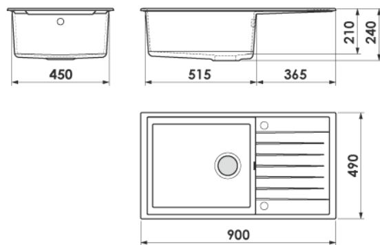
DŘEZ S ODKAPEM pravý / levý číslo modelu: 229 rozměr: 90cm x 49cm
